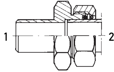
Zayıflatıcı Rakor Adaptör Reducing Union Adaptor
