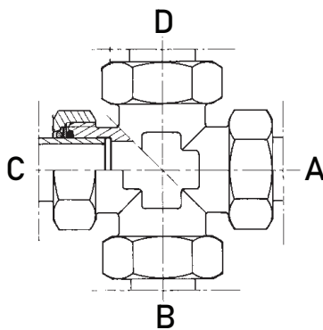
Basınç Düşürücü Kros Reducing Cross
