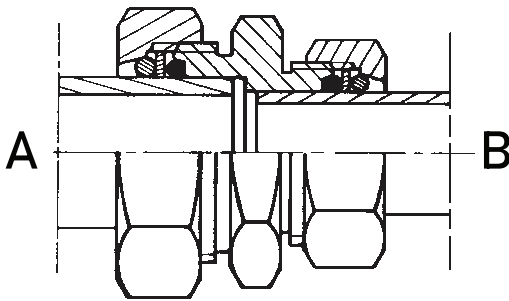
Paralel Erkek Bağlantı Reducing Union
