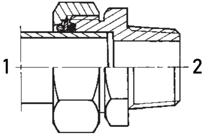
Paralel Erkek Bağlantı Parallel Male Union
