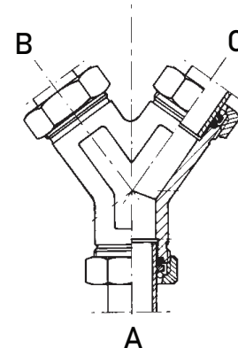
Basınç Düşürücü Y Reducing Y Branch
