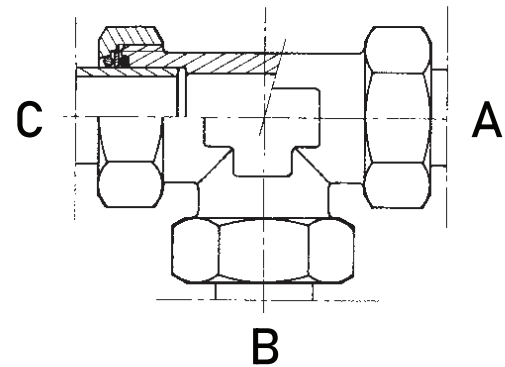
Basınç Düşürücü T Reducing Tee
